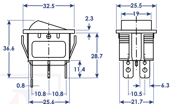
fig. Rocker Switch
